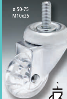
RUOTA CON SUPPORTO ROTANTE A CODOLO FILETTATO
