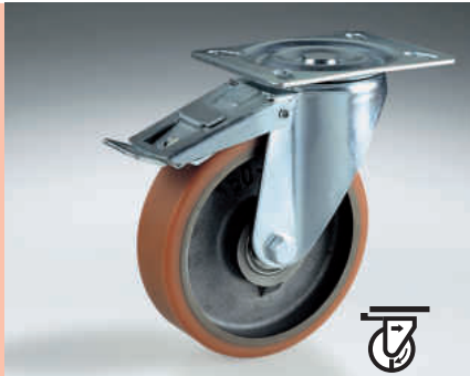
RUOTA CON SUPPORTO ROTANTE A PIASTRA CON FRENO TOTALE ANTERIORE
