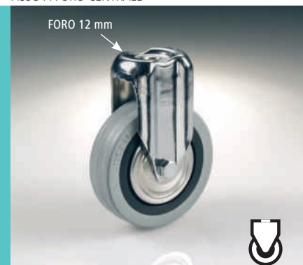
RUOTA CON SUPPORTO FISSO A FORO CENTRALE
